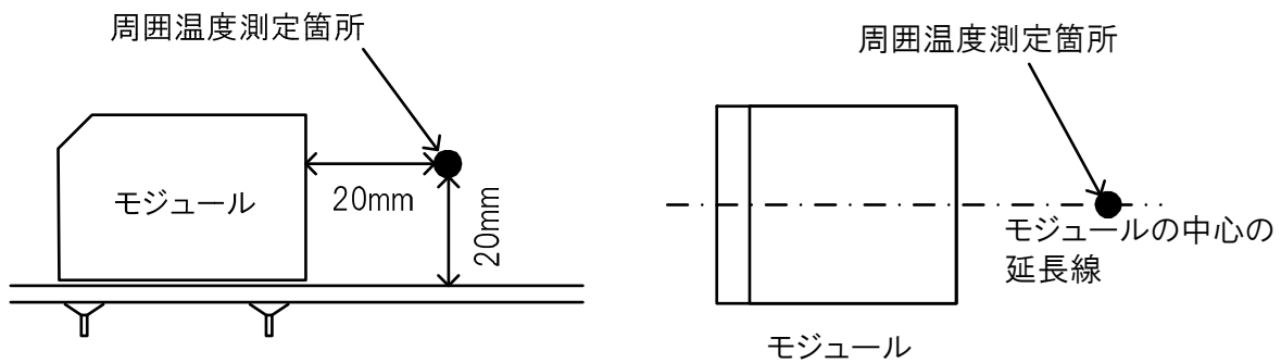
発熱部品の影響がない場合の周囲温度測定箇所
